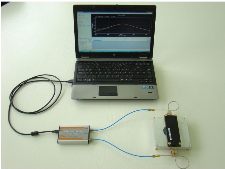
Fotografia zestawu mikrofalowego do bezkontaktowego pomiaru rezystywności/rezystancji na kwadrat metodą dielektrycznego rezonatora postumentowego
